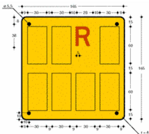
Figura III.4/n Art. 258 - Targa di prova - Figura III.4/s Art. 258
