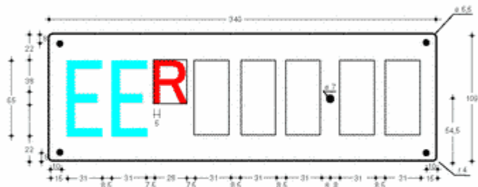
TARGA RIPETITRICE PER VEICOLI TRAINATI DA AUTOVEICOLI "ESCURSIONISTI ESTERI"
