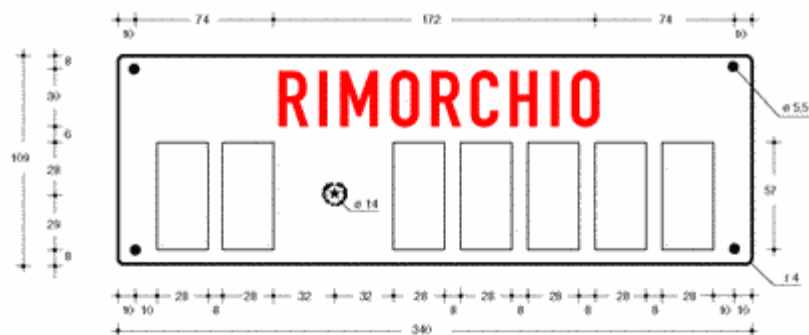
Figura III 4/d Art. 258 TARGA DI IMMATRICOLAZIONE DEI RIMORCHI DEGLI AUTOVEICOLI
